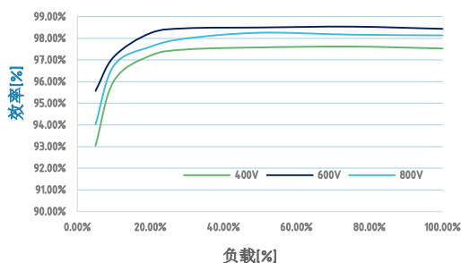
效率曲线
