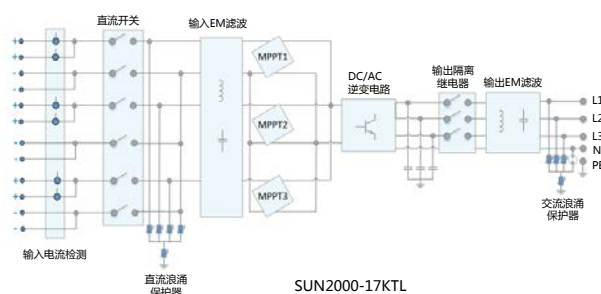
电路框图
